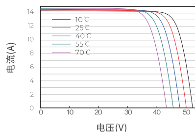
电流-电压曲线 JAM72S30-575/LR
