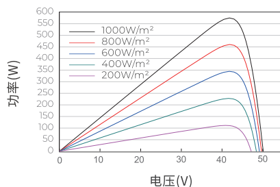
功率-电压曲线 JAM72S30-575/LR
