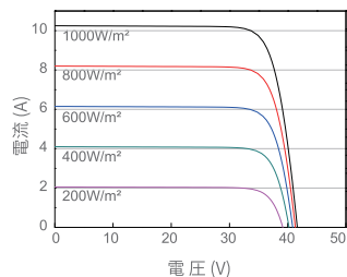
電流-I-Vカーブ JAM60D10-340/MB
