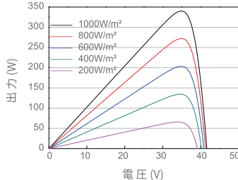
出力-I-Vカーブ JAM60D10-340/MB
