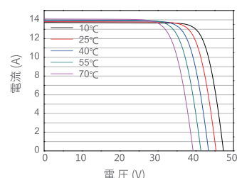
電流-I-Vカーブ JAM66D30-495/MB
