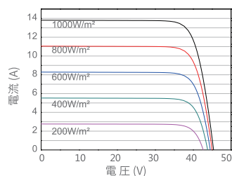
電流—I-Vカーブ JAM66D30-495/MB
