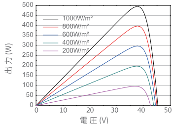
出カーI-Vカーブ JAM66D30-495/MB
