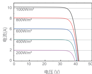
电流-电压曲线 JAM60D10-340/MB
