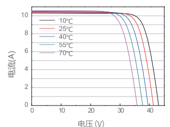
电流-电压曲线 JAM60S10-335/MR
