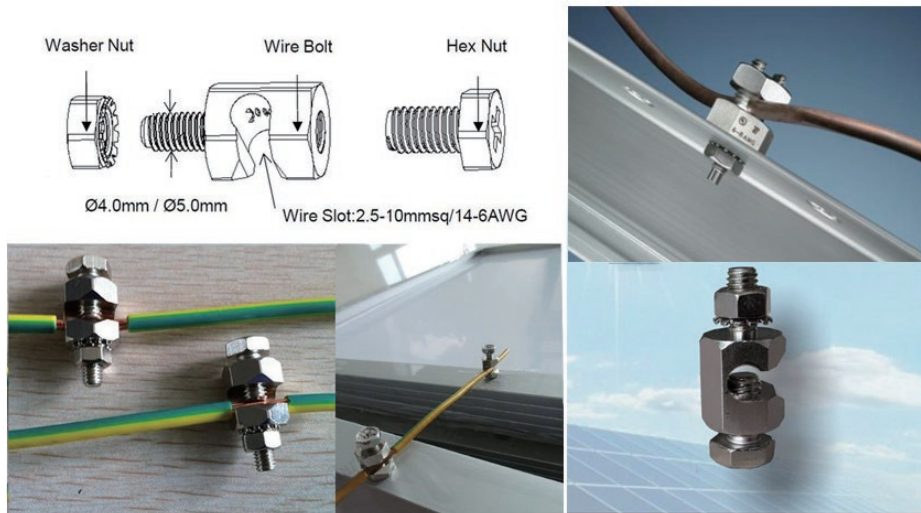
图6 接地方式
