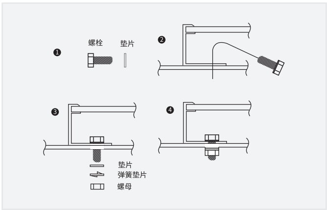
图2安装方式
